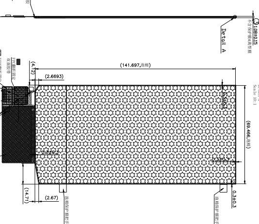
侧视图
