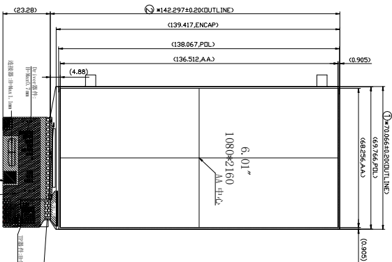
正视图
